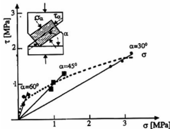
Hình 3 - Đồ thị phân tích thí nghiệm cắt biến góc
