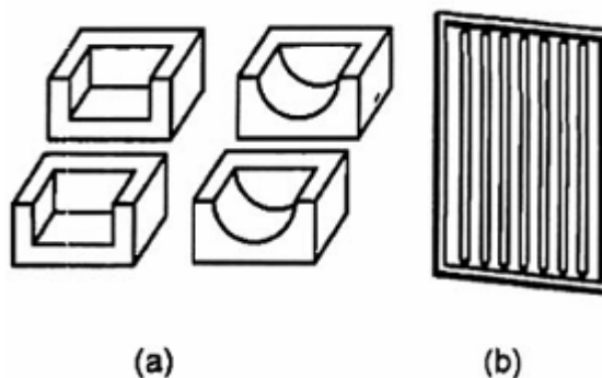
Hình 5 - Bộ khuôn giữ mẫu và hệ thống con lăn
