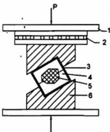
Hình B1 - Sơ đồ thí nghiệm cắt biến góc trên mẫu bán quy cách
